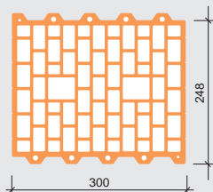
Przekrój pustaka Porotherm 30 E3
