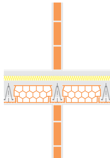
ściana Porotherm 8 P+W / Profi / Dryfix
